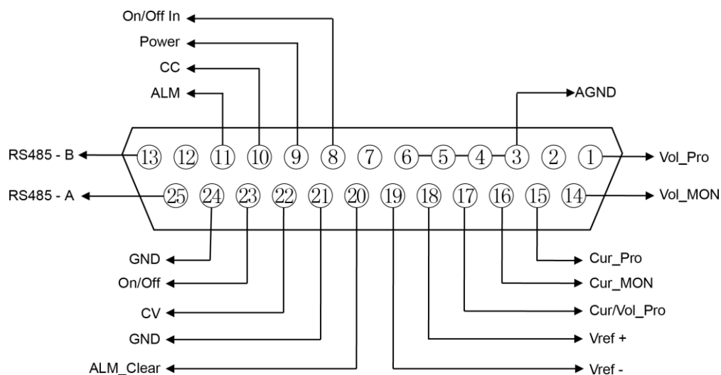
図 7-1 DB25外部アナログ制御ユニット
