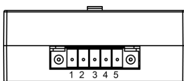
RS-232各ピン
